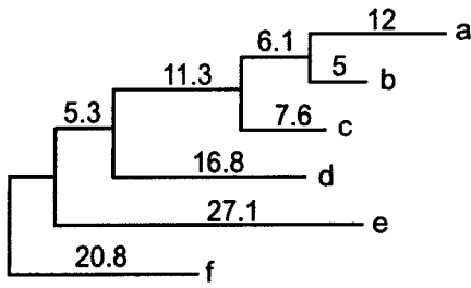
(D) Maximum parsimony tree
